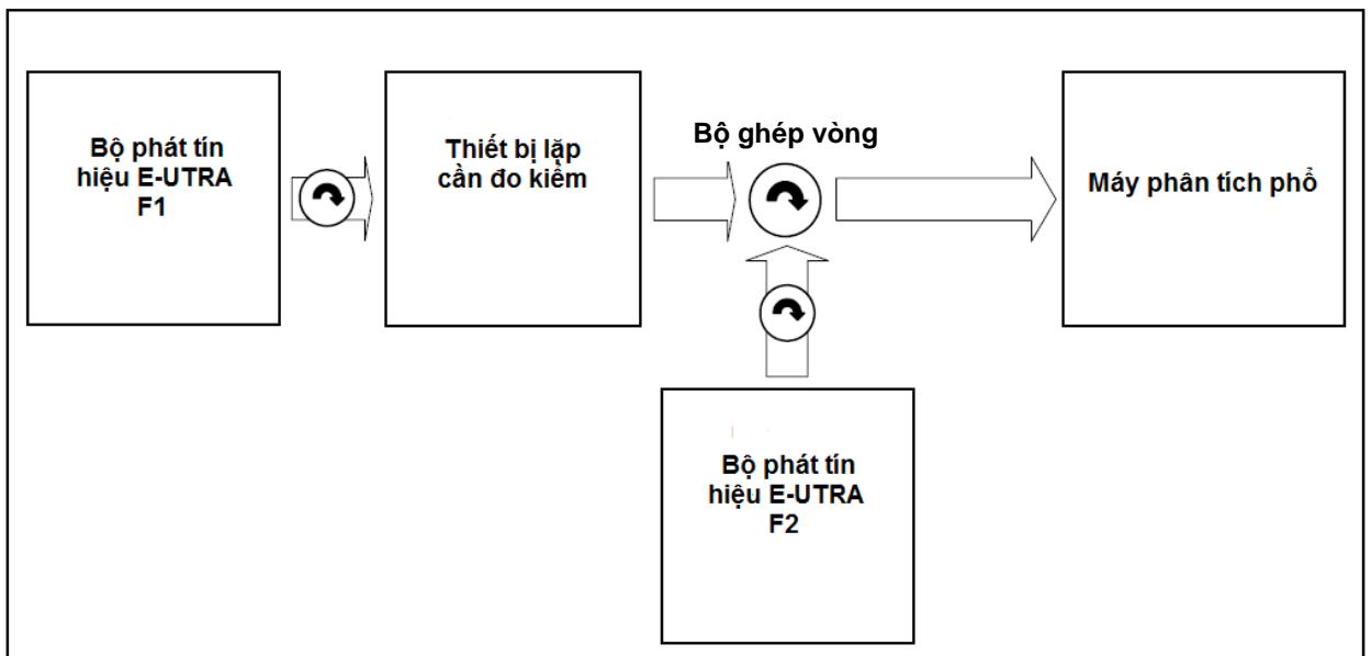
Hình C. 6 – Sơ đồ hệ đo xuyên điều chế đầu ra
