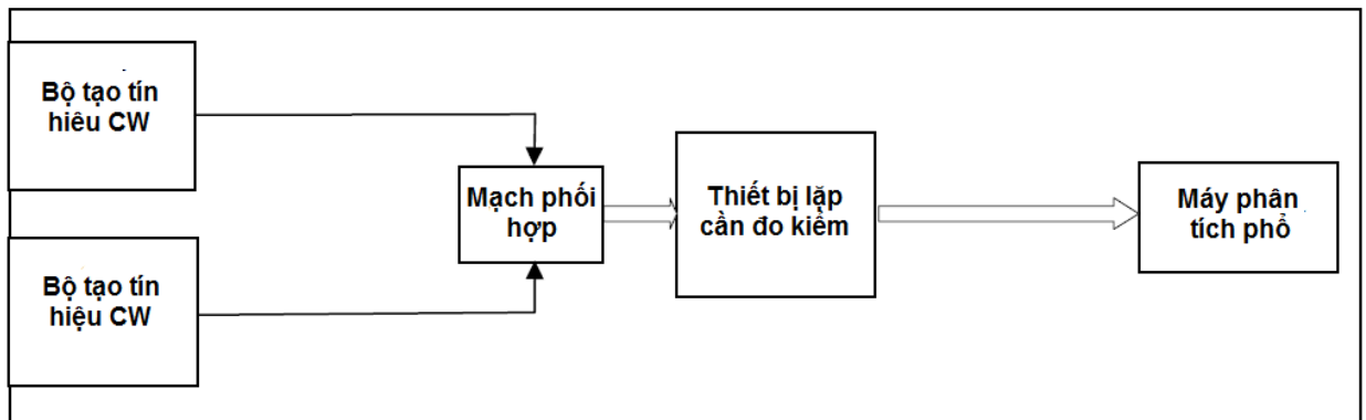
Hình C. 5 – Sơ đồ hệ đo xuyên điều chế đầu vào
