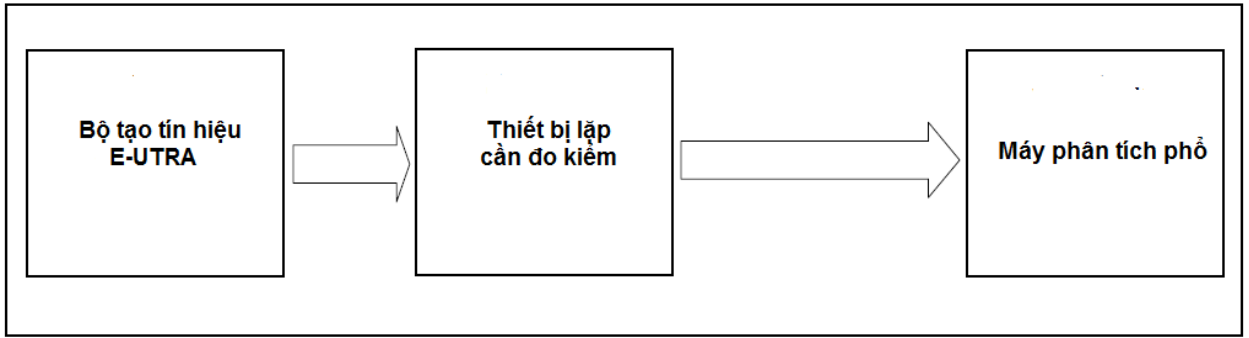
Hình C. 4 – Sơ đồ hệ đo phát xạ không mong muốn: Phát xạ giả
